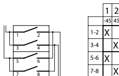
Przelącnik 1-2 (schodowy)
