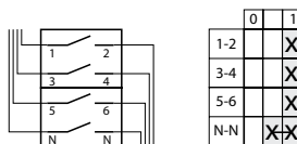
Przelącnik 1-2 (krzyżowy)
