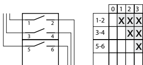
2.8445 Łącznik obwodów 0-1-2-3
